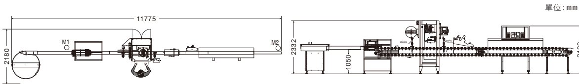
機械尺寸圖
