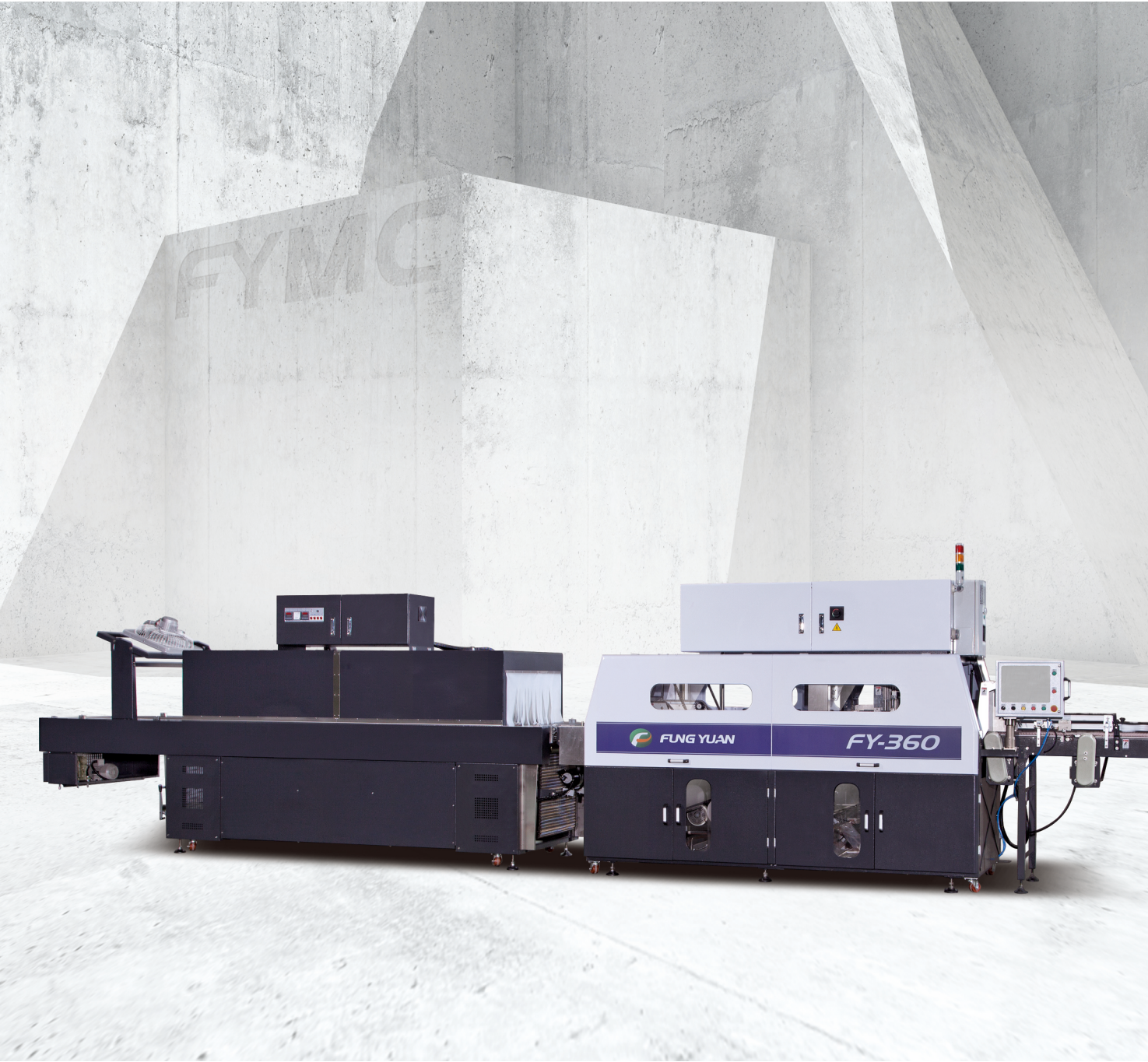
底部搭接式收縮膜包裝，適用於 400~500 BPM 的產線。
