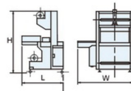
機械尺寸圖 M / C Dim. Illustration
